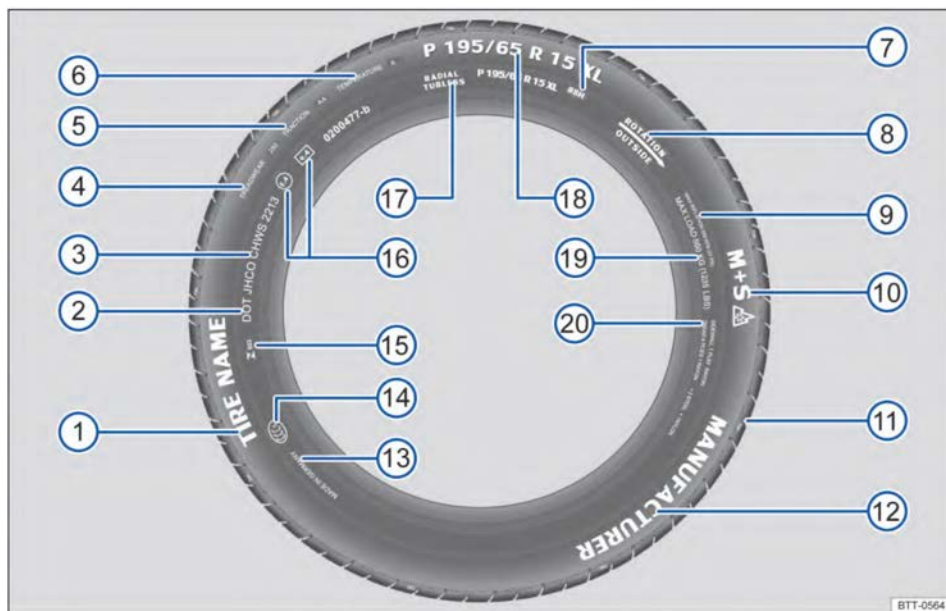
تصویر ۱۹۴ کد بین‌المللی شناسایی لاستیک
