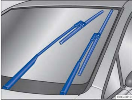
تصویر ۱۶۳ برف پاک‌کن شیشه جلو در وضعیت سرویس و نگهداری
