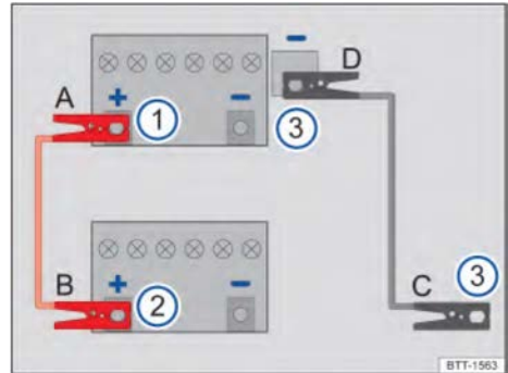
تصویر ۱۷۱ تصویر اتصال کابل‌های باتری به باتری
