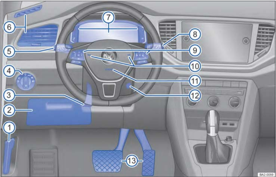
تصویر ۷ نمای کلی داخل کابین سمت راننده (T-Roc)
