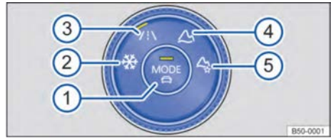
تصویر ۱۰۹ قسمت پایین داشبورد: کلید کنترل فعال 4MOTION برای مدل‌های 4WD
