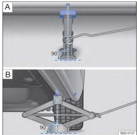
تصویر ۲۰۰ نقطه حمایت جک
