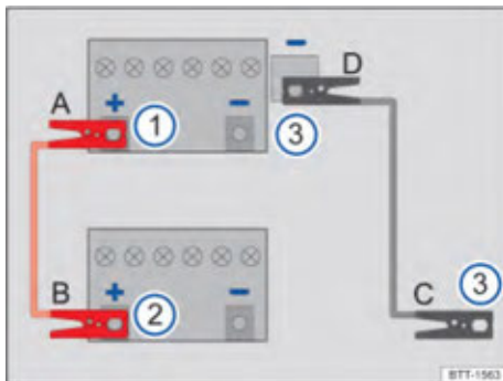
تصویر ۱۵۵: تصویر اتصال کابل‌های باتری به باتری
