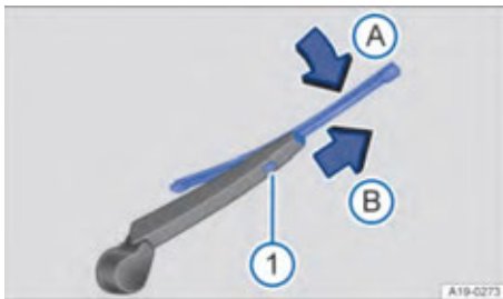
تصویر ۱۴۹: تعویض تیغه برف پاک‌کن شیشه عقب
