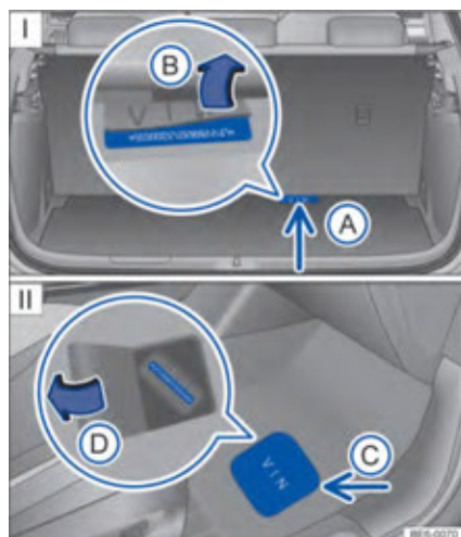
تصویر ۱۸۵: شماره شناسایی خودرو (VIN): ① روی پنل کف عقب خودرو (تیپ I); ② روی پنل کف سمت سرنشین جلو (تیپ II)
