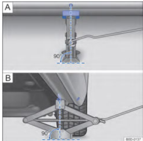
تصویر ۱۷۵: جک در قسمت عقب سمت چپ خودرو قرار گرفته است.
