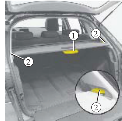
برای باز کردن طاقچه عقب بخش متحرک
