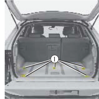
نقاط دارای قلاب داخل صندوق
